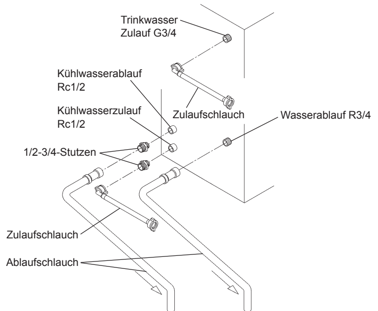
Wassergekühltes Modell [b] (IM-45WNE/65WNE)
