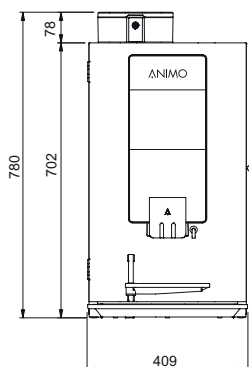
VOORAANZICHT
